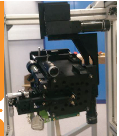
Projet SKYDICE : système de calibration photométrique basé sur des LEDs.
