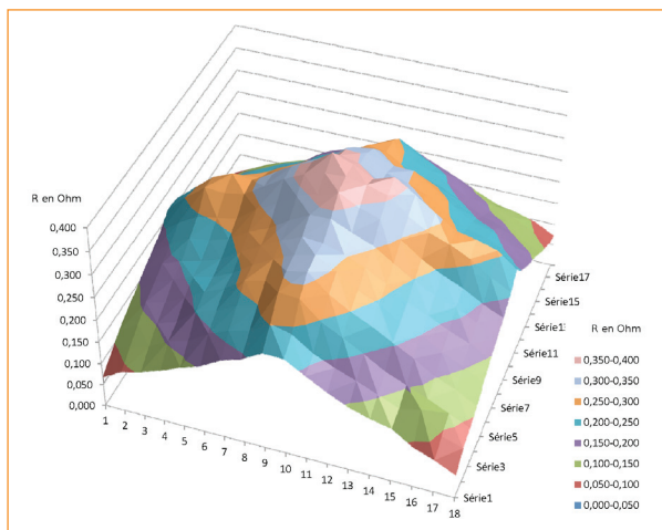
Mesure des résistances de contact sur une éprouvette de la taille d'un capteur silicium pour le projet ILD/CALICE.
