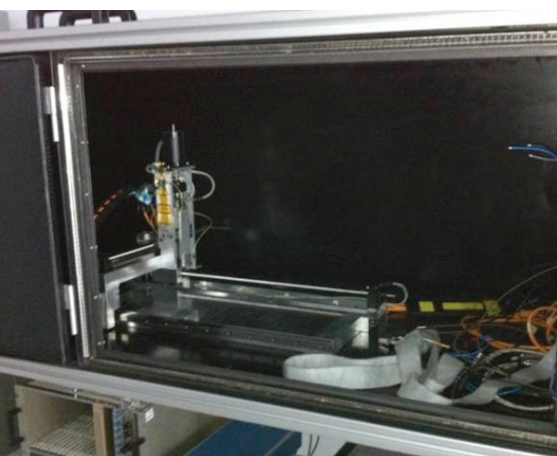
Cage de Faraday dans la salle de test ATLAS.
