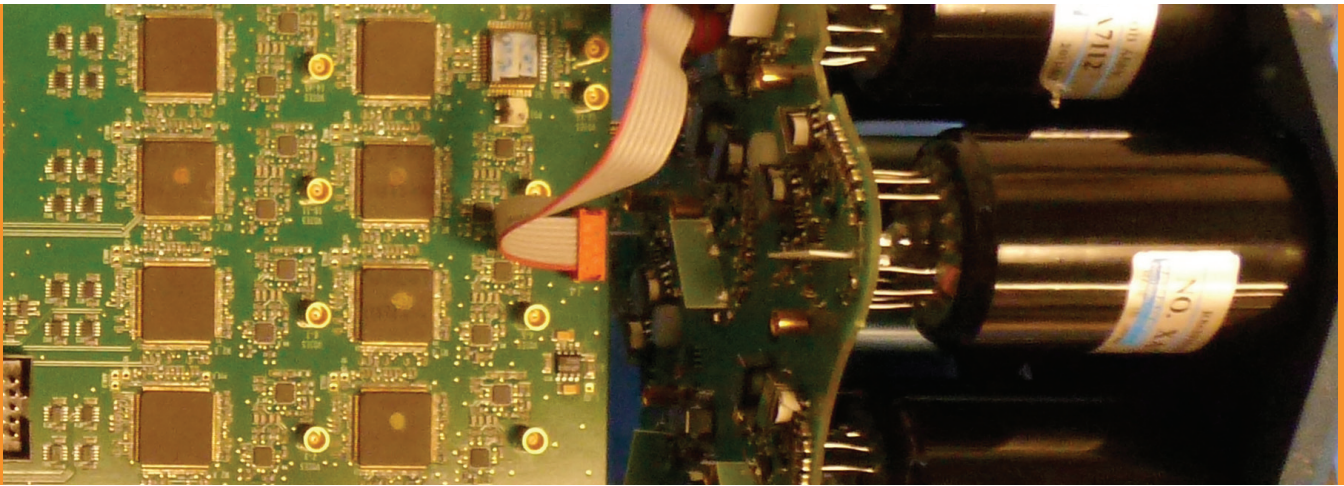
Le module NeCTAr pour le projet CTA.
