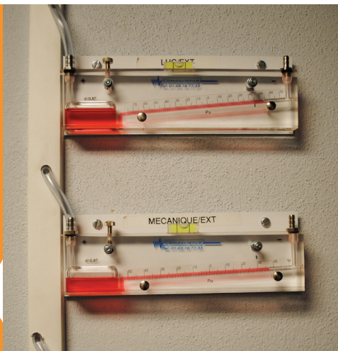
Manomètres à colonnes en entrée de salle propre (suivi des cascades de pression).
