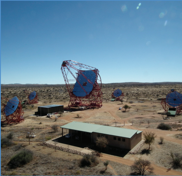
La caméra HESS II au milieu des 4 caméras HESS I.
