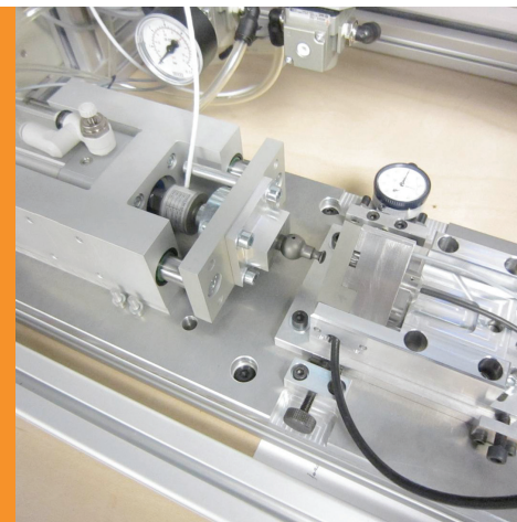
Banc de test du système de verrouillage pour le projet LSST.
