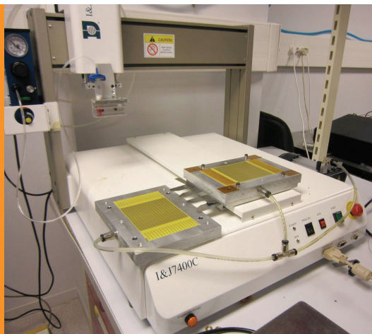
Robot de collage pour les détecteurs du projet ILD/CALICE.
