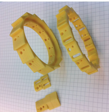
Anneau support pour la couche supplémentaire autour du beam pipe d'ATLAS.
