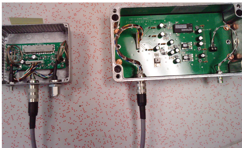
Carte d'alimentation pour les antennes décamétriques du projet AUGER.
