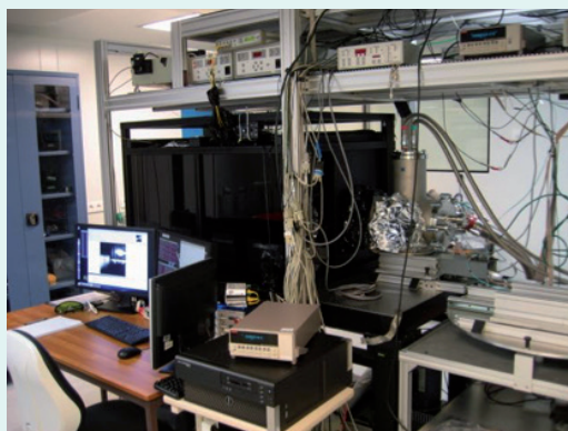
Banc CCD complètement équipé avec l'électronique de lecture de LSST.
