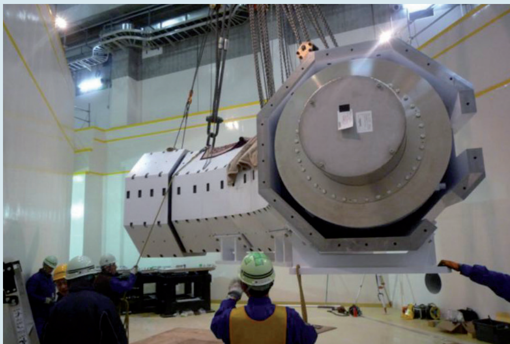
Installation de l'aimant de transport des muons dans le Hall COMET à J-PARC.
