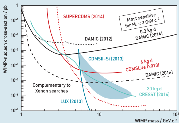
Courbes d'exclusion à 90 % de niveau de confiance pour différentes expériences. La courbe DAMIC-100 est une projection basée sur l'exposition de 100 g de CCD pendant 1 an (30 kg.day) avec un bruit de fond limité à 0.3 dru (0.3 événement par keV/kg/day au dessus de 50 eV).
