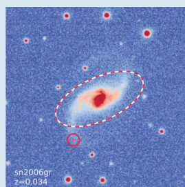
Galaxies hôtes des supernovae de type Ia SN2006gr (SDSS) et 04D2bt (SNLS) obtenues dans la bande optique g et situées respectivement à un redshift de 0.034 et 0.22.
